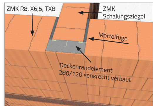
Ansicht Detail
